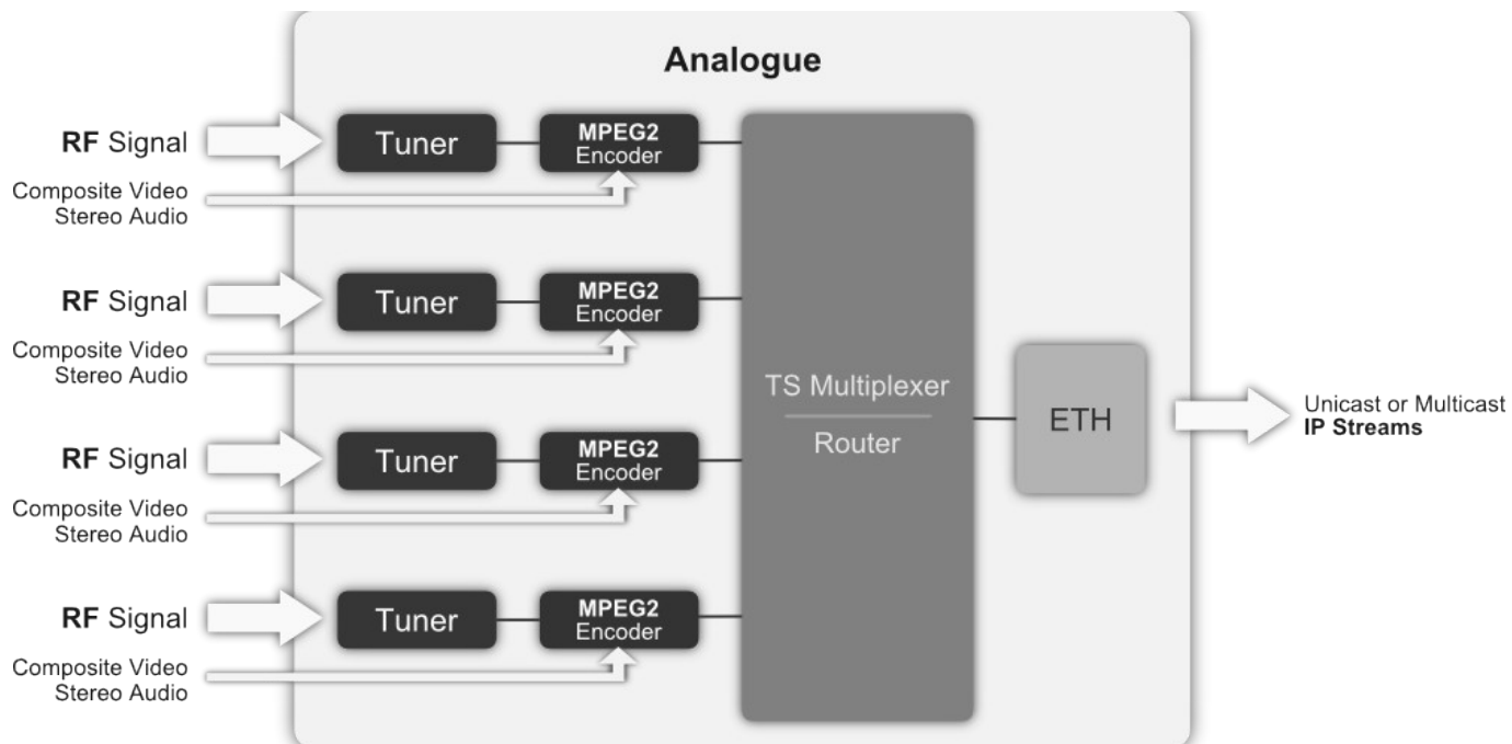
A Nowision Receiver belső blokkvázlata
